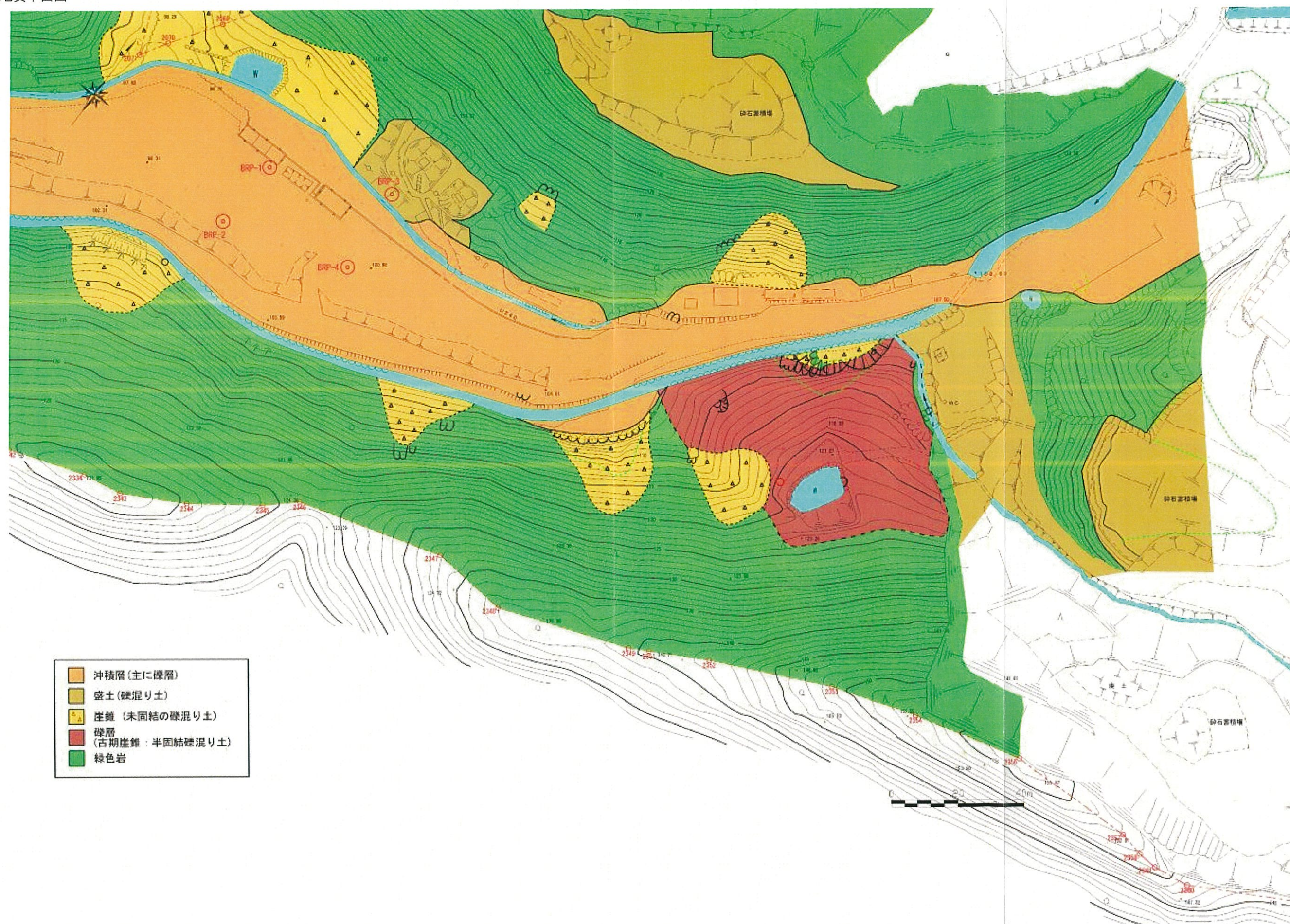
図 1.6 地質平面図
